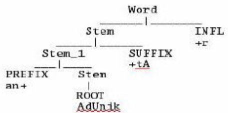
Figure 2: Parse tree for “anAdUniktAr” (অনাদুনিকতার)
